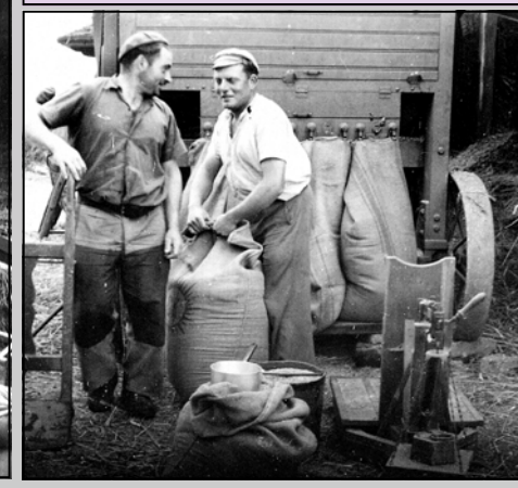
Photos de la batteuse en activité dans la vallée du Boulon.
